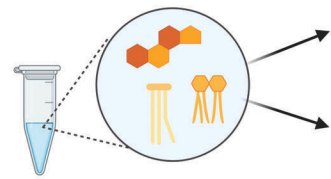
ANALIZA LIPIDOMICZNA
