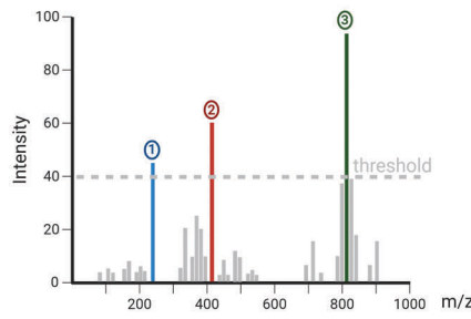
ANALIZA PROTEOMICZNA
