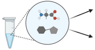
ANALIZA METABOLOMICZNA
