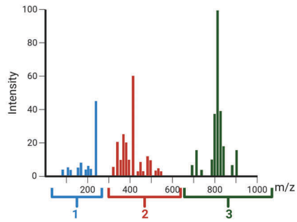
ANALIZA METABOLOMICZNA
