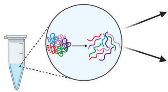
ANALIZA PROTEOMICZNA
