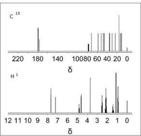
NMR
