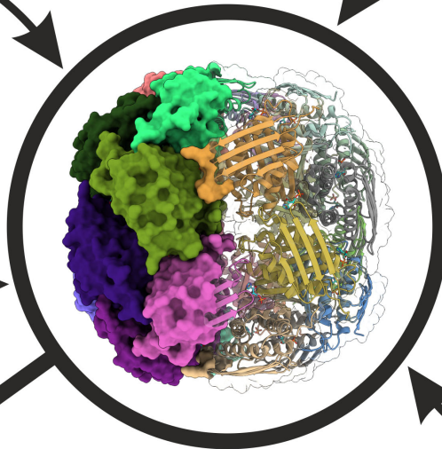
Biocząsteczki
