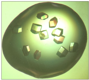
Krystalografia
